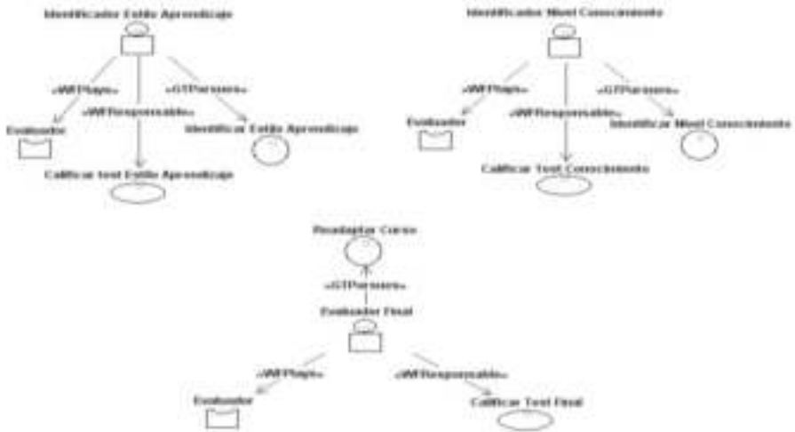
Figura 5.3. Modelo de agentes con INGENIAS
