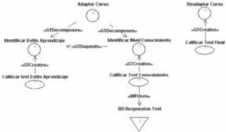
Figura 5.4. Modelo de tareas y objetivos con INGENIAS
